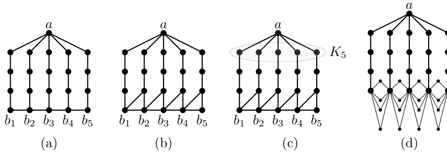
Fig. 5. (a) X_k (b) Y_k (c) Z_k (d) W_k .
